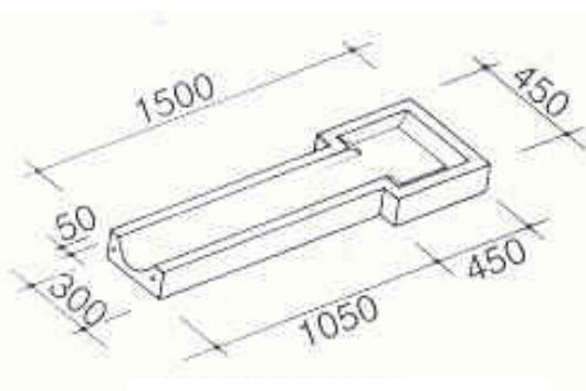
Loiskekivi LK 300
