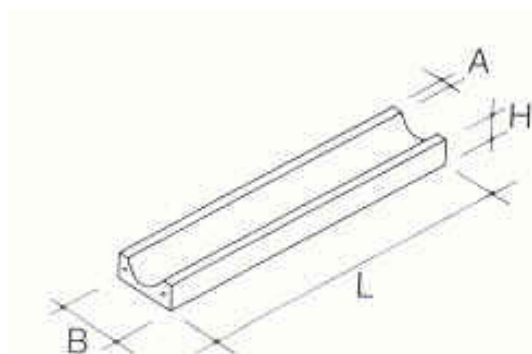
Vesikouru VK 260 - 400
